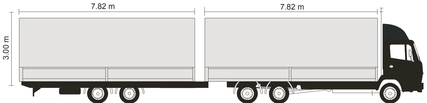
Kurzkoppelfahrzeug
